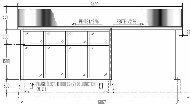
Élévation principale
