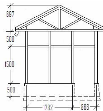
Élévation (porte)
